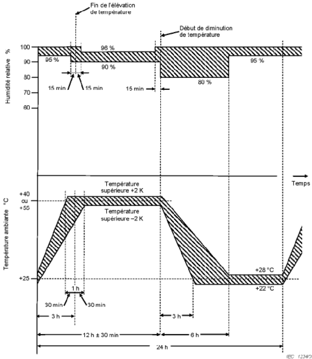
Figure 2b -Essai Db - Cycle d'essai - Variante 2
